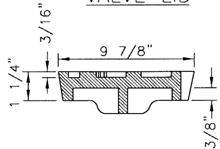
PROFILE VALVE LID
