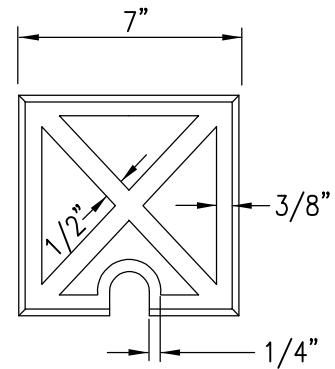
LID BOTTOM PLAN
