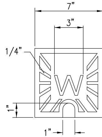
LID TOP PLAN
