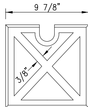
LID BOTTOM PLAN
