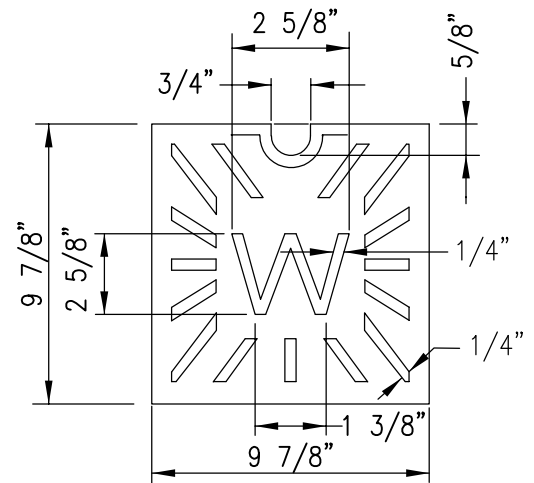
LID TOP PLAN
